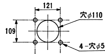
取付穴詳細図
