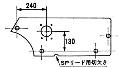
取付穴位置
