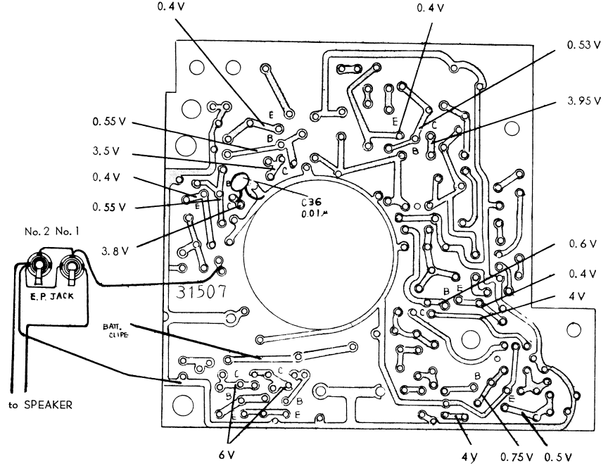
7TA-4型 サークिटボード裏面図
