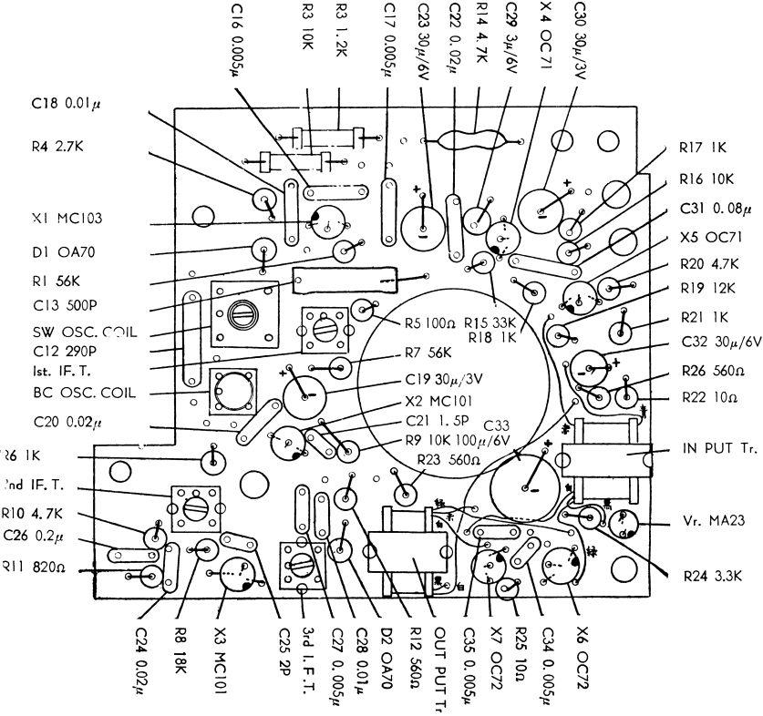
7TA-4型 部品配置図
